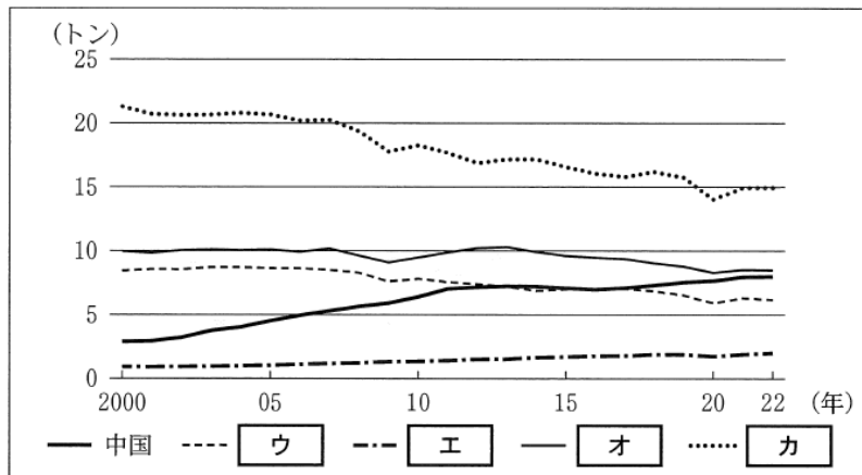
図 2-2 二酸化炭素の一人当たり排出量
